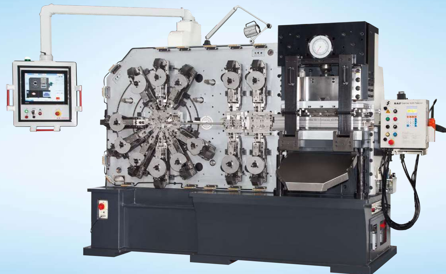
可選用全伺服滑座 OPTIONAL: SERVO DRIVEN SLIDE
